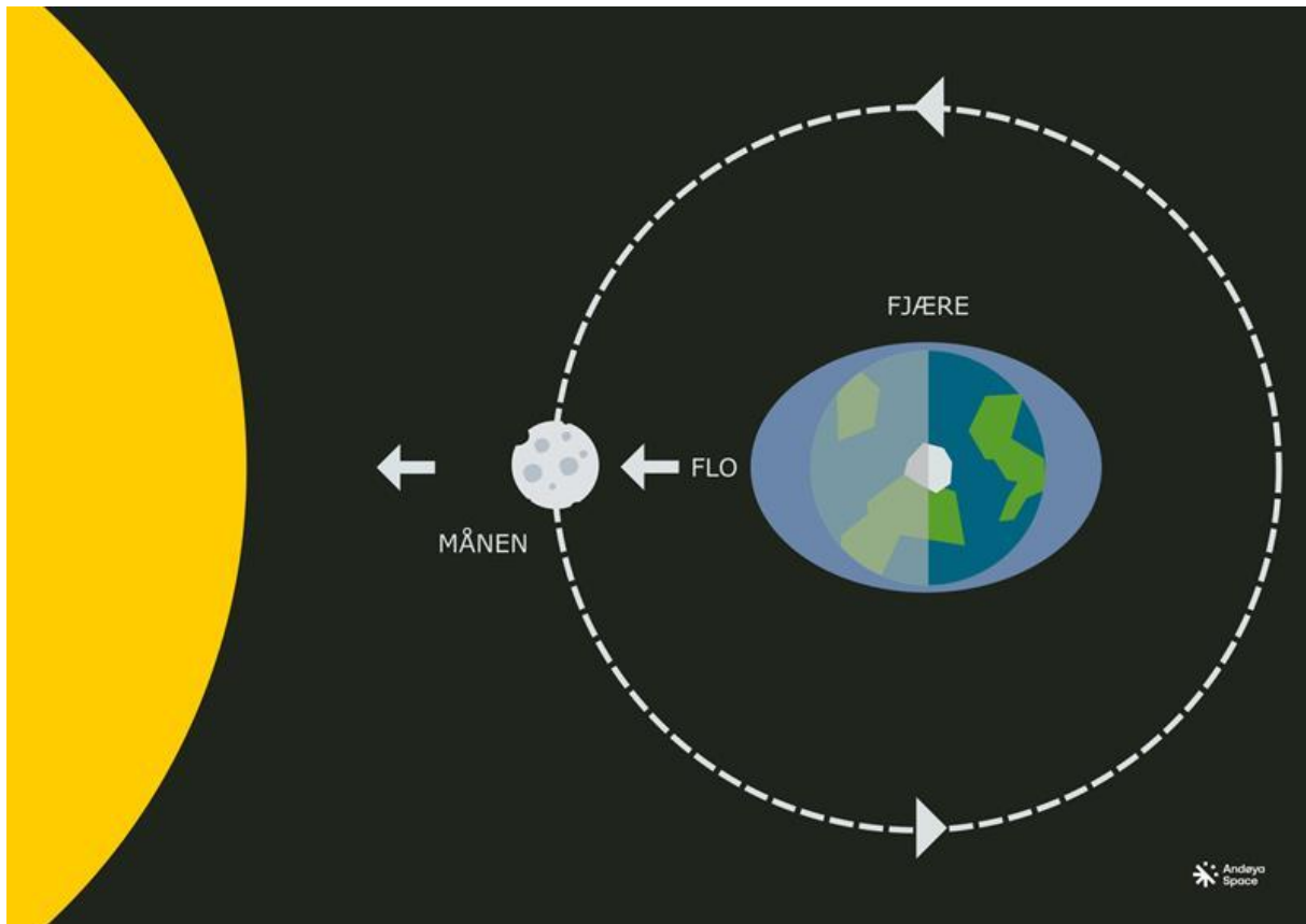
Figur 3: Månen og tidevannet. Illustrasjon av Andøya Space Education
