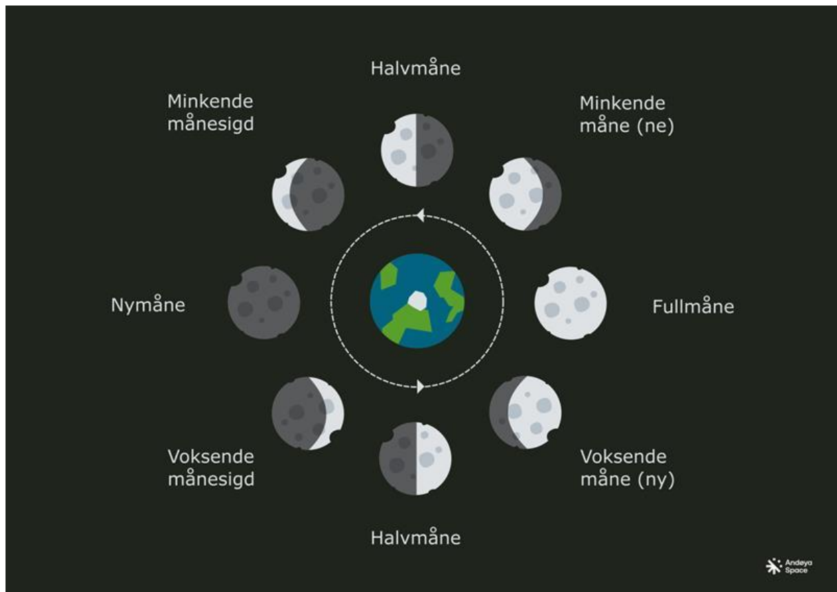
Figur 1: Månefasene. Illustrasjon: Andøya Space Education
