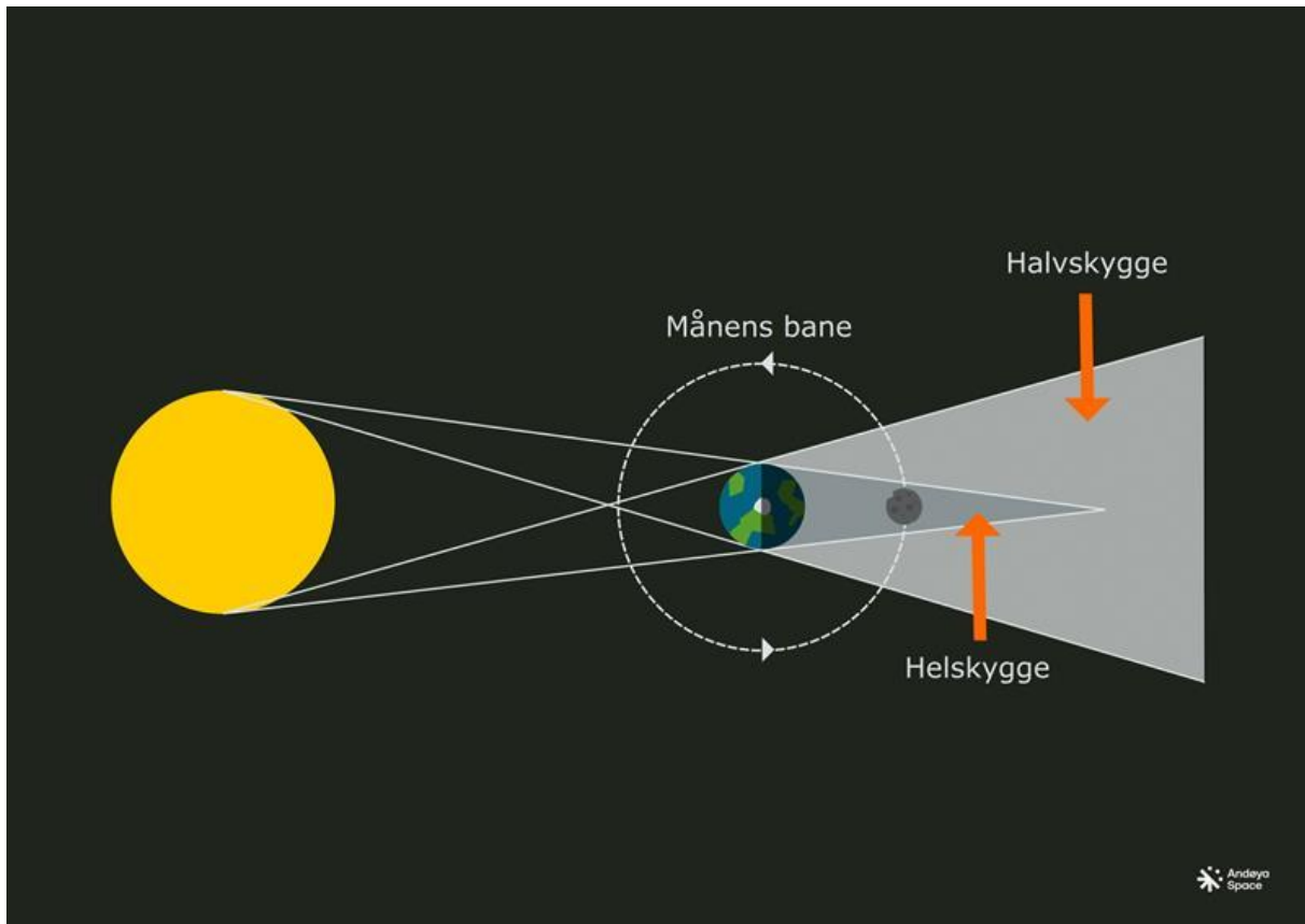
Figur 2: Måneformørkelse. Illustrasjon: Andøya Space Education
