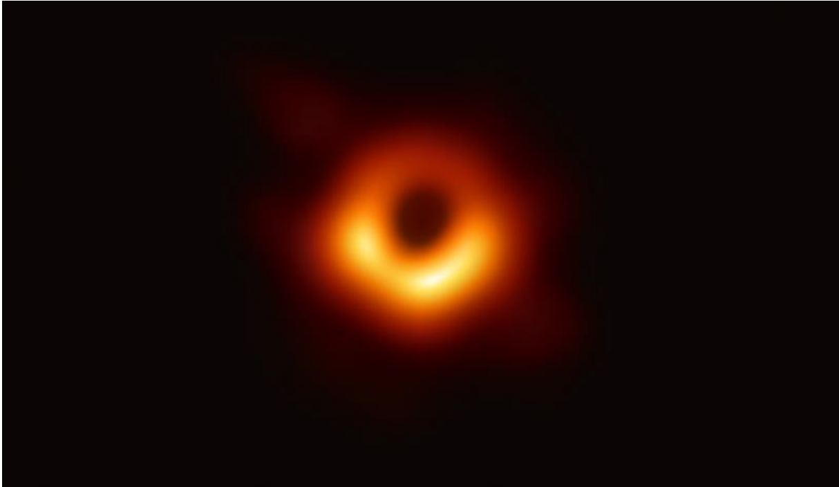
Figur 1: Det første faktiske bilde av et svart hull i galaksen M87. Kilde: NASA/Event Horizon Telescope collaboration et al.
